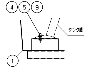
A-A 断面詳細図 S=1/10
