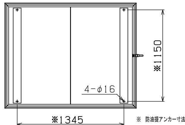
底面図
