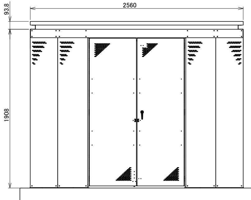
承認図
